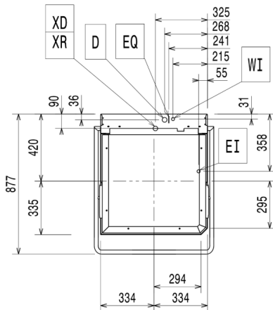
Päältä
