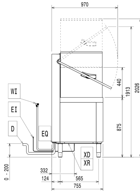
Sivulta
